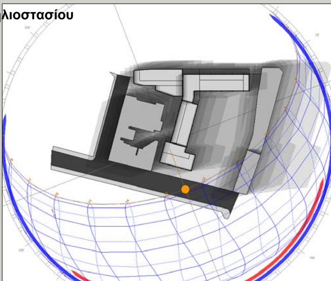
Εύρος σκίασης κτηρίου την ημέρα του θερινού ηλιοστασίου
