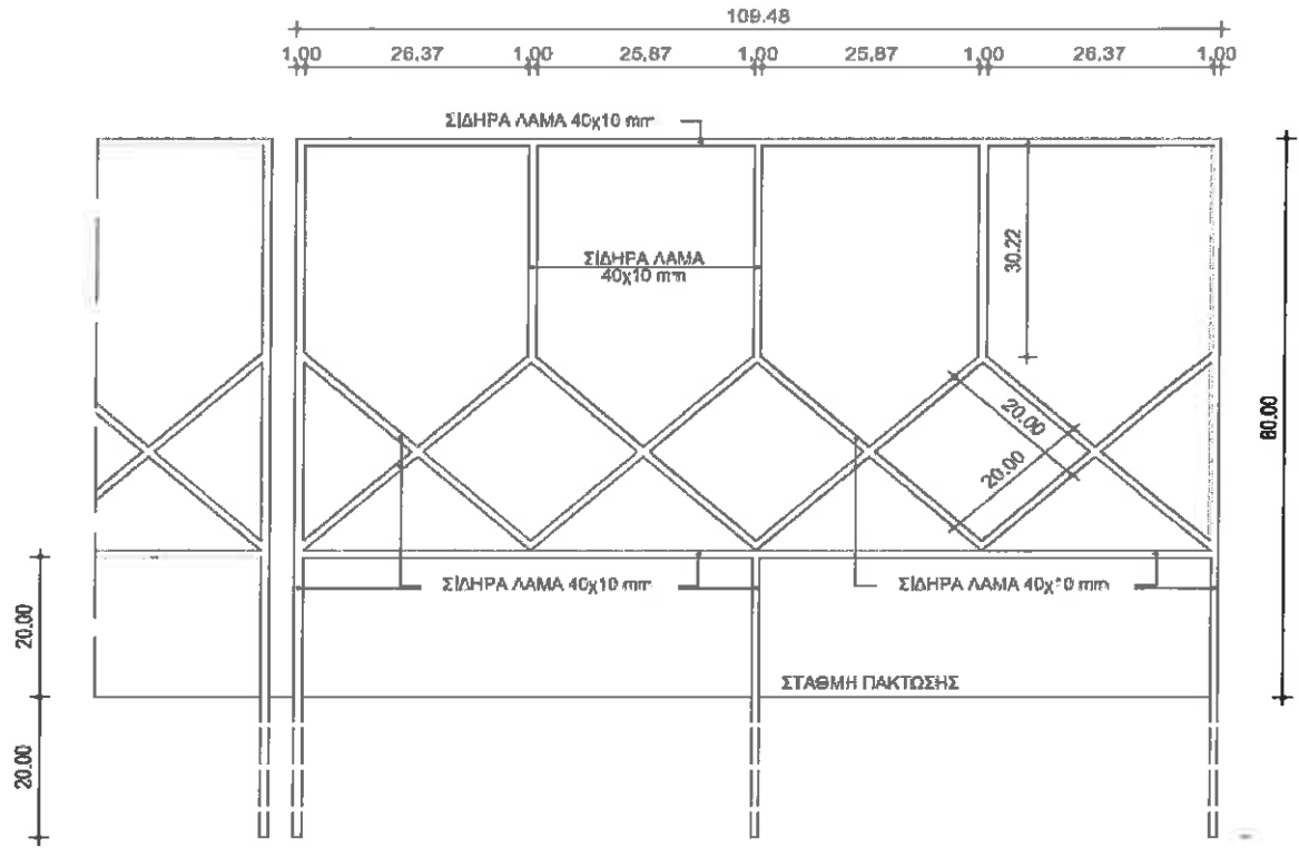
ΚΛΙΜΑΚΑ 1:4
