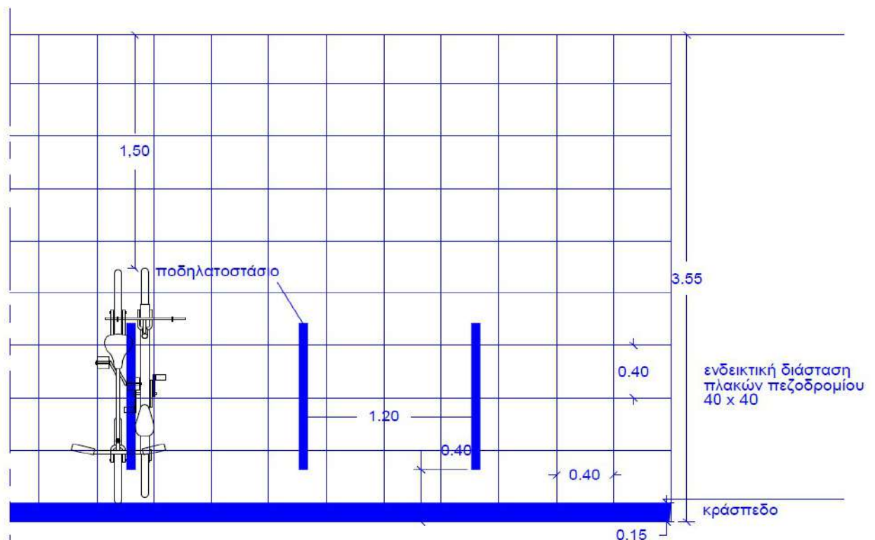
Σχέδιο 4: Κάθετη τοποθέτηση ποδηλατοστασιων
