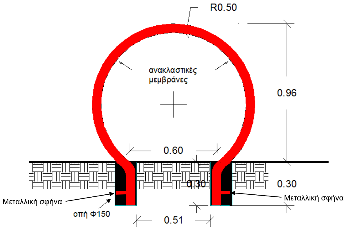
Σχέδιο 2: Σχήμα και Διαστάσεις ποδηλατοστάσιου
