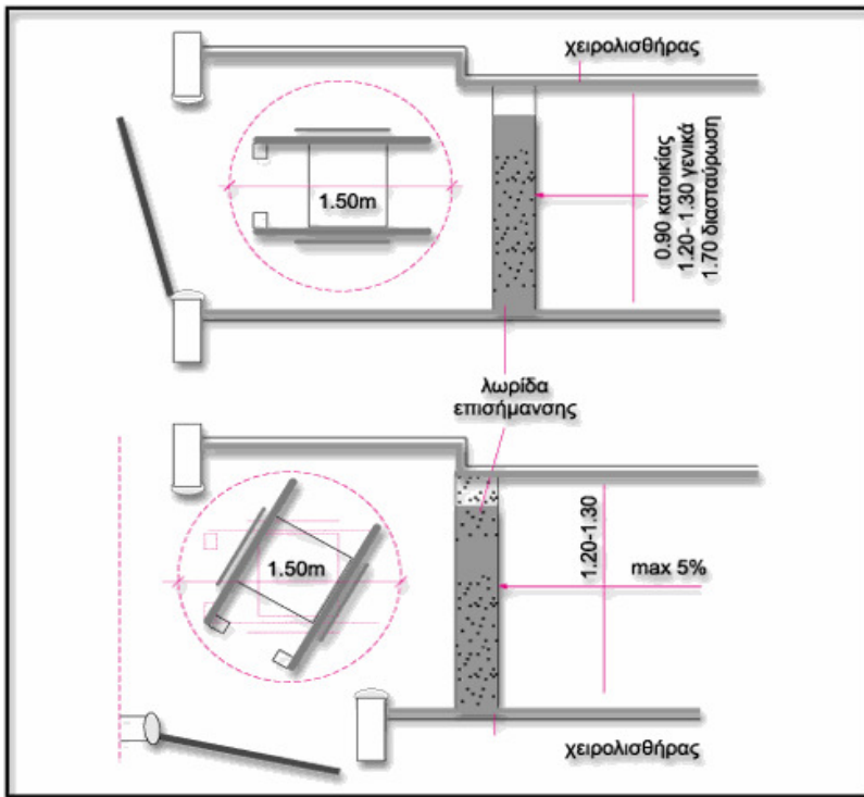
Κατασκευή ράμπας με πλατύσκαλο
