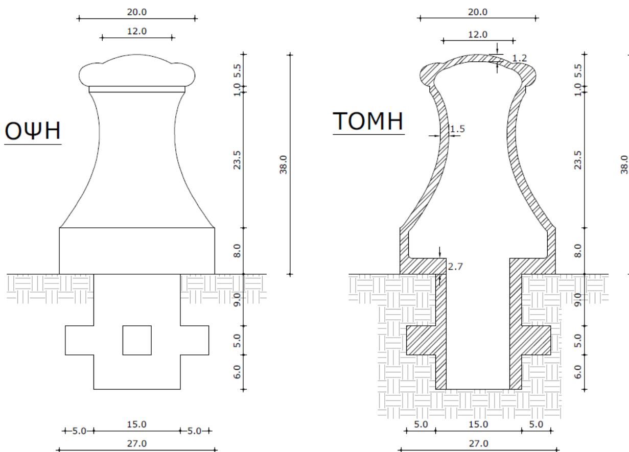
ΑΠΟΤΡΕΠΤΙΚΟ ΧΥΤΟΣΙΔΗΡΟ ΕΜΠΟΔΙΟ ΤΥΠΟΥ ΔΕΣΤΡΑΣ
