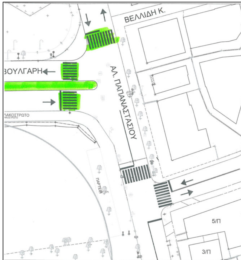
Εικόνα 7: Κόμβος Αλ.Παπαναστασίου – Αγησιλάου - Βούλγαρη
