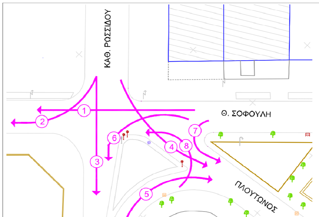
Εικόνα 5: Κινήσεις νόμιμες και παραβατικές στον κόμβο Θ.Σοφούλη-Καθ.Ρωσσίδου
