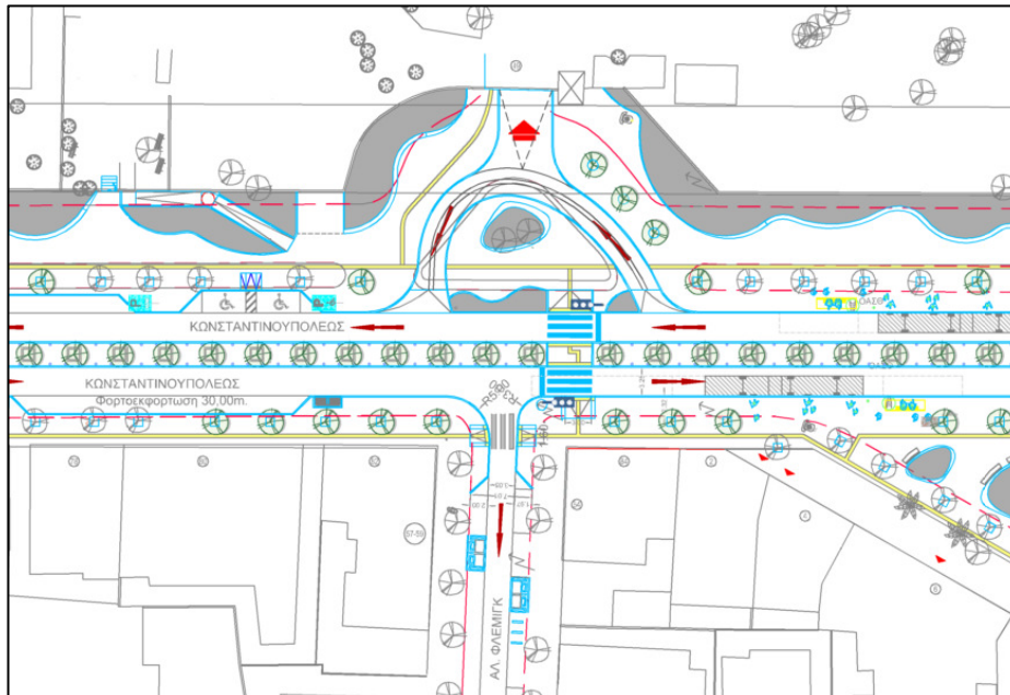
Εικόνα 1: Κωνσταντινουπόλεως – είσοδος Ιπποκράτειου
