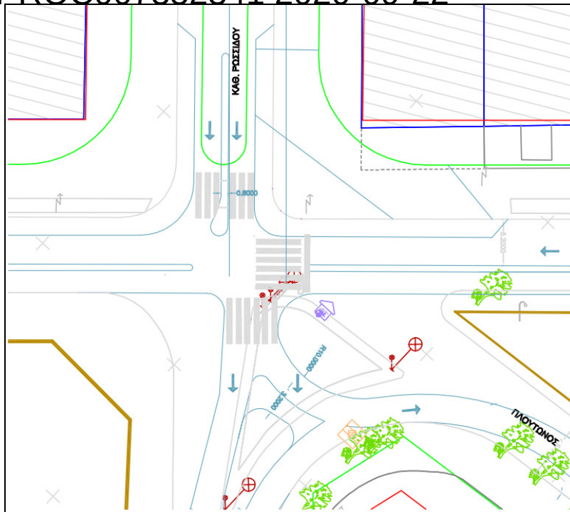
Εικόνα 6: Ανασχεδιασμός Κόμβου Θεμ.Σοφούλη – Καθ.Ρωσσίδου
