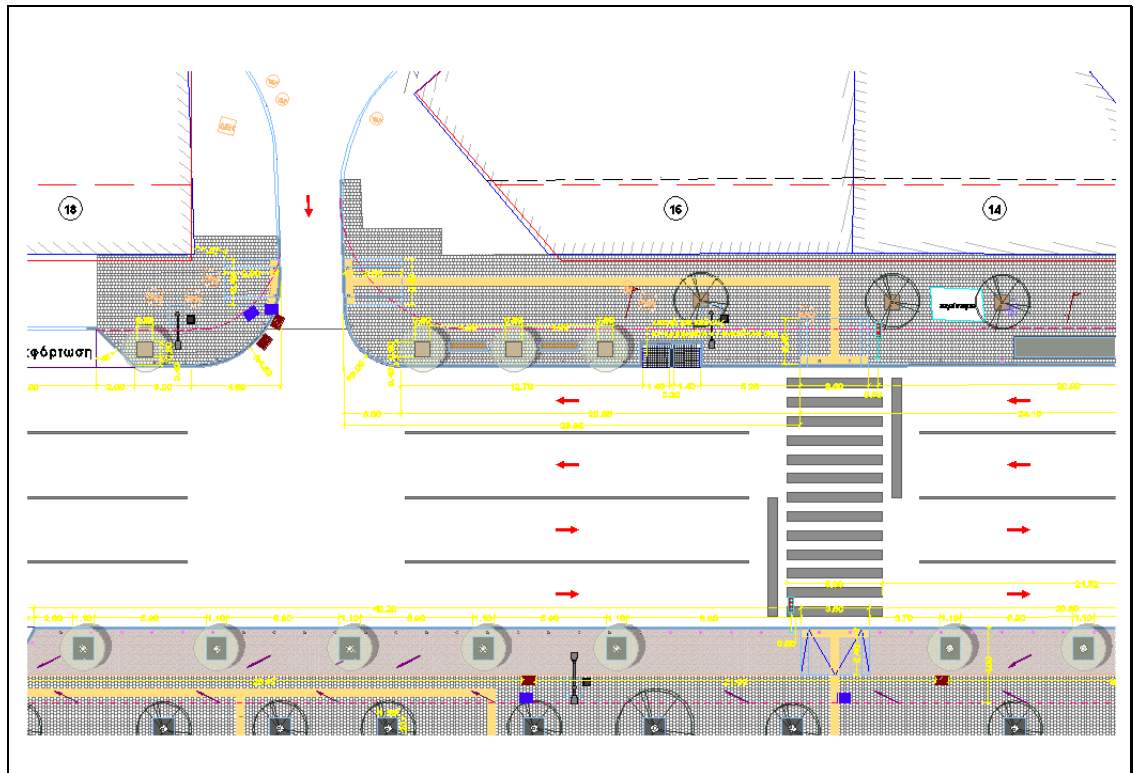
Εικόνα 2: 26 ης Οκτωβρίου – είσοδος Δικαστηρίων
