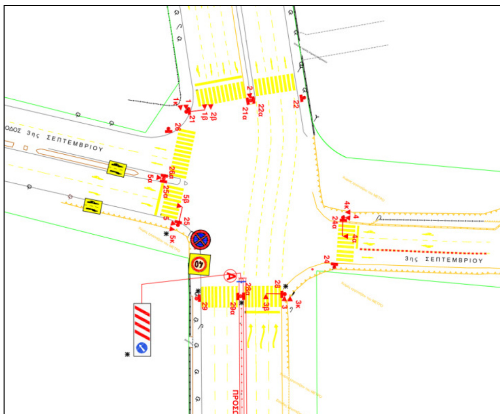
Εικόνα 3β: Εγνατία – 3ης Σεπτεμβρίου
