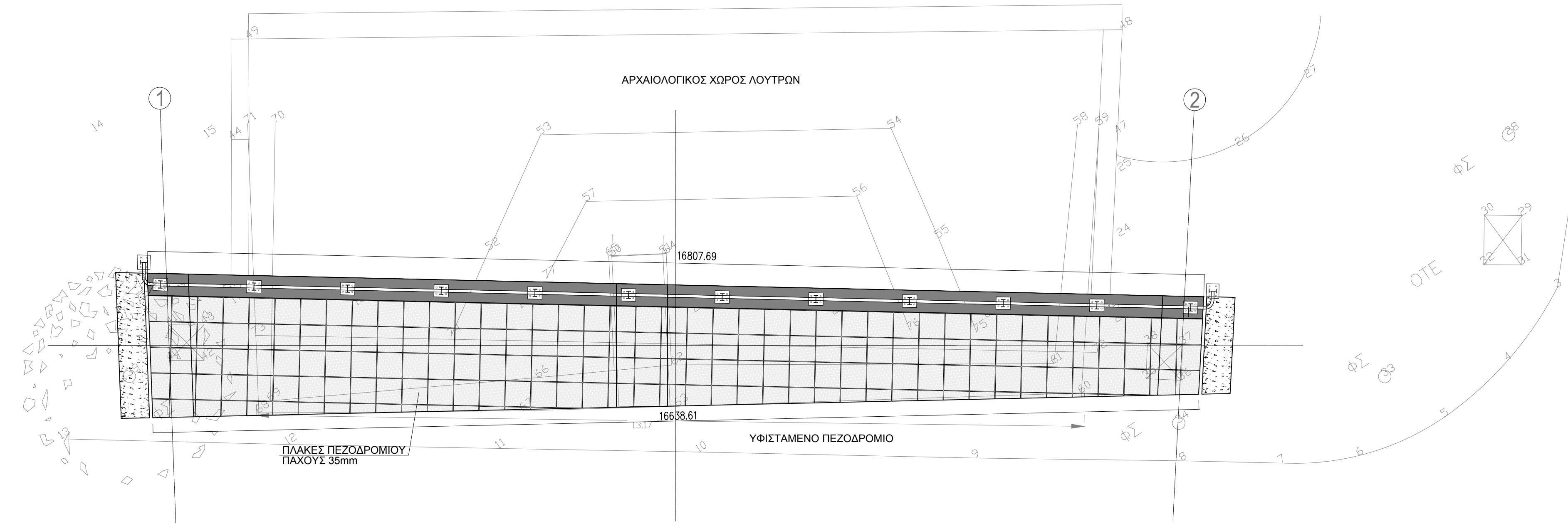
ΚΑΤΟΨΗ ΠΕΖΟΓΕΦΥΡΑΣ ΚΛ. 1:50
