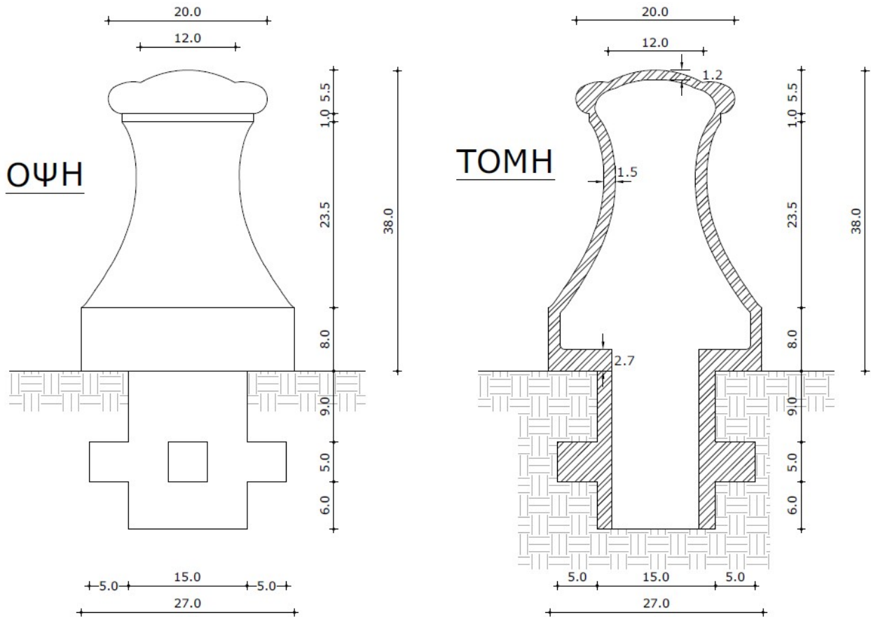
ΑΠΟΤΡΕΠΤΙΚΟ ΧΥΤΟΣΙΔΗΡΟ ΕΜΠΟΔΙΟ ΤΥΠΟΥ ΔΕΣΤΡΑΣ
