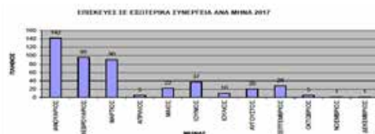
Διάγραμμα 2: Εισερχόμενες βλάβες που προορίζονται σε εξωτερικά συνεργεία ανά μήνα για το έτος 2017
